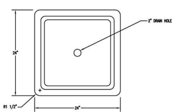
1 TOP VIEW Scale: 1/8" = 1"
